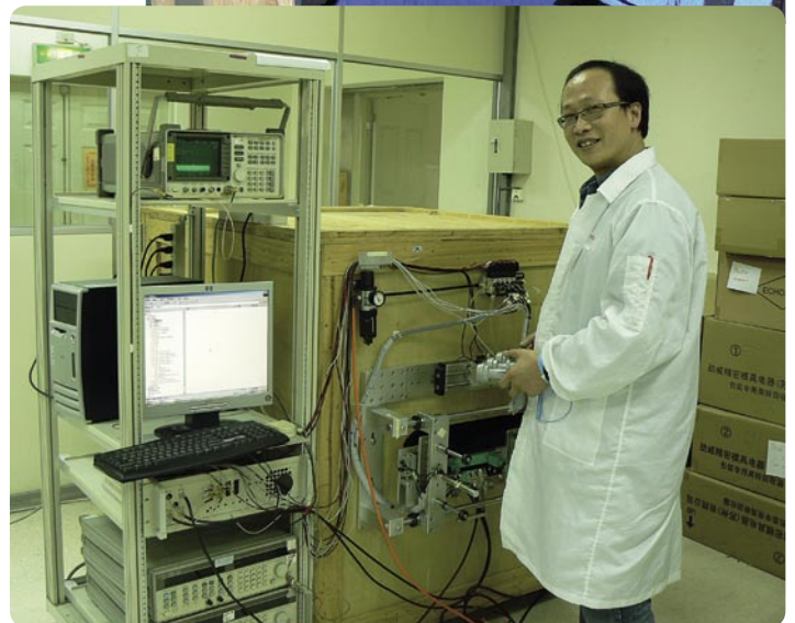
Pan Yuonan ürün geliştirme mühendislerinden biri. Burada yeni geliştirilmiş üçlü bir LNB'nin yankısız odada çapraz modülasyon direncini test ediyor. Test odasının iç kısmı yukarıdaki resimde açık kapıdan görülebilir.
